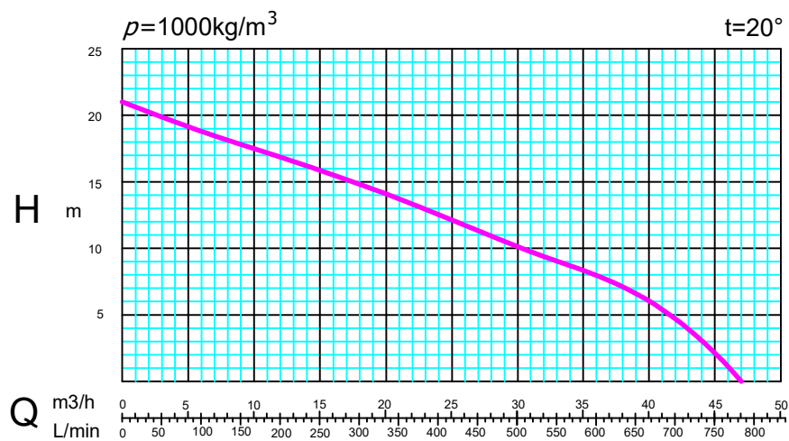
Характеристики погружного насоса
